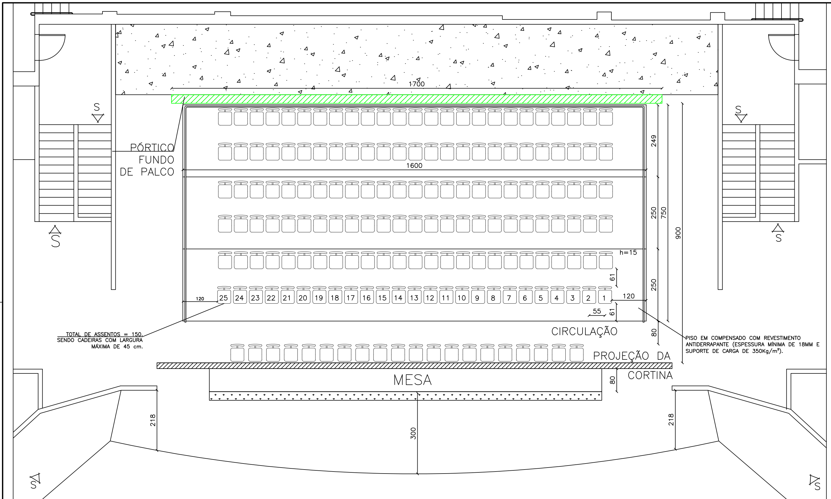
DETALHE PALCO ESCALA 1:75
